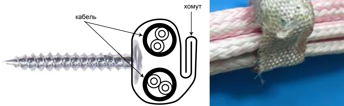
Рис. 7. Установка дюбель–хомута КФСТ.735322.041. Вариант 3.
