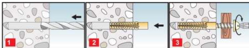
Рис. 2. Установка дюбеля КФСТ.735322.095 и КФСТ.735322.096.
