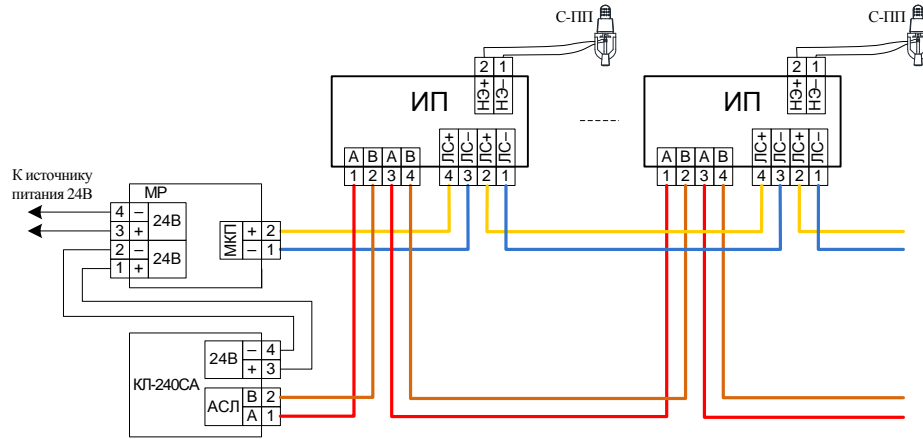
Рисунок 1 – Схема подключения извещателей.
