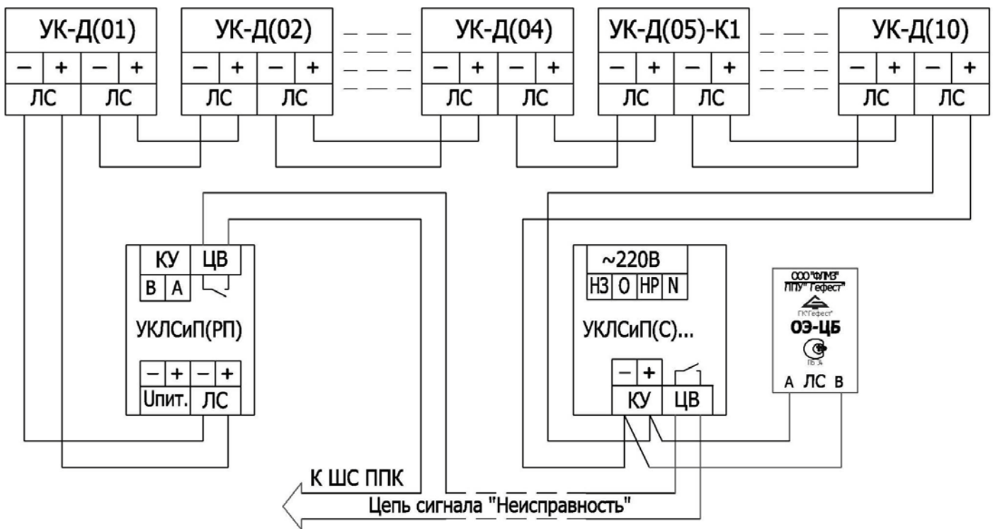
Рис.4 Схема подключения к ЛС УКЛСиП(РП) устройств УК-Д(01)...УК-Д(10) и УКЛСиП(С)
