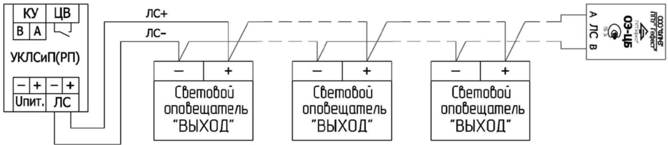
Рис.1 Схема подключения световых оповещателей в режиме постоянного свечения (команда "Пуск" на УКСиП(РП) не подается)
