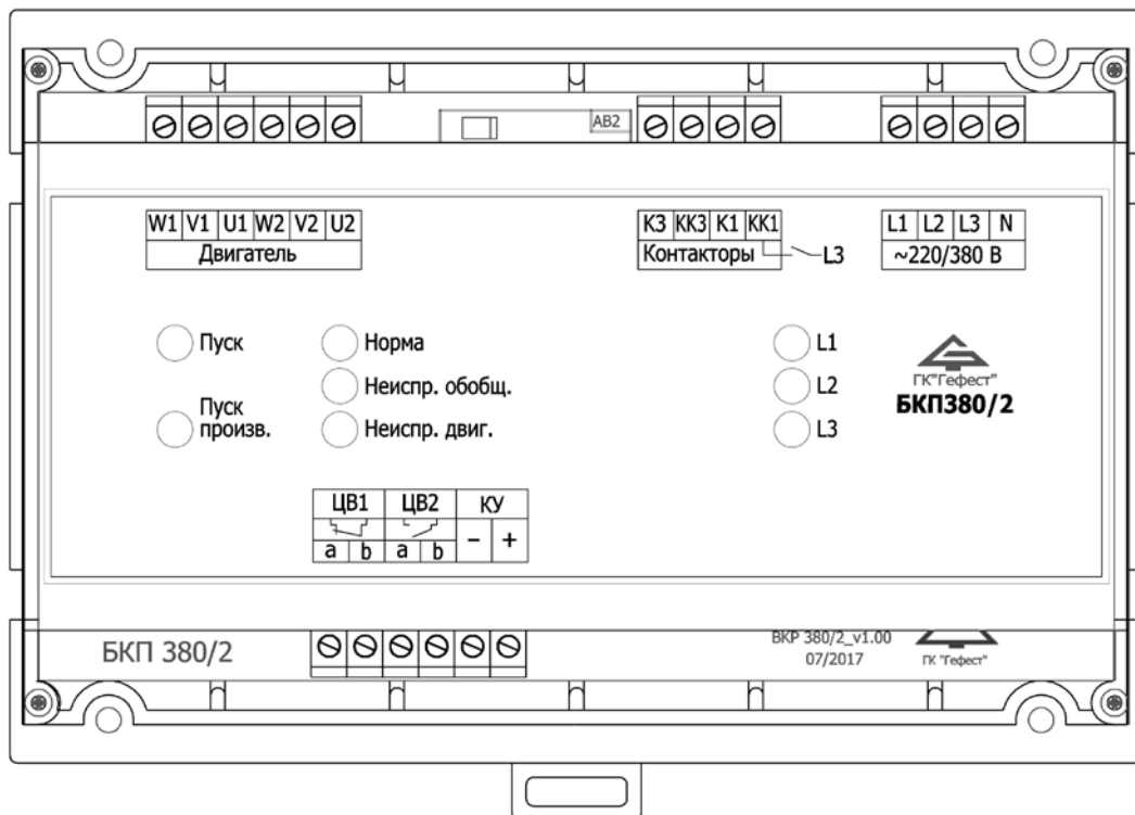
Рисунок 1 – Внешний вид БКП380/2
